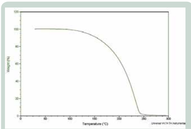
热重分析（TGA）采取的升温速度为10°C/分钟。
